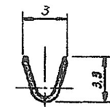
断面 B-B
